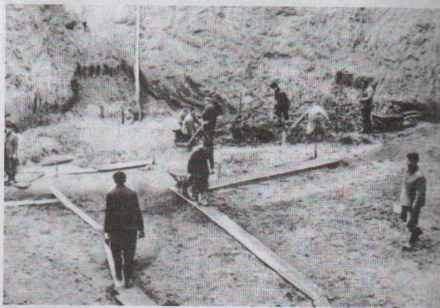
Budowa wymagająca prowadzenia głębokich prac ziemnych
